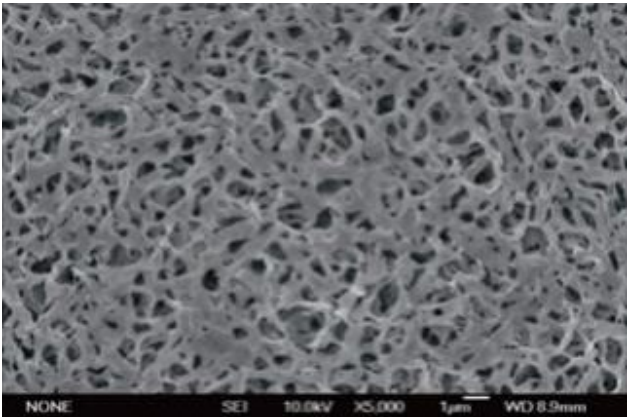
亲水 PVDF 膜 (0.22μm) 的 扫描电镜照片
